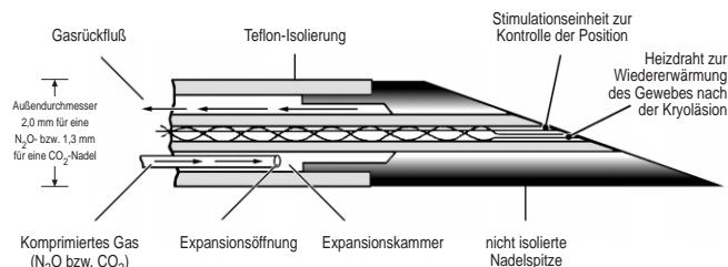
Abb. 5 Schematischer Längsschnitt durch eine Punktionsnadel zur Durchführung der Kryoanalgesie mit N_2O ; bei den CO_2 -Kryosonden ist die Nadelspitze gerundet
