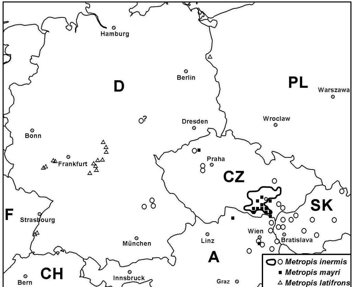
Abb. 2: Fundorte der Arten der Gattung Metropis in Mitteleuropa nördlich der Alpen
